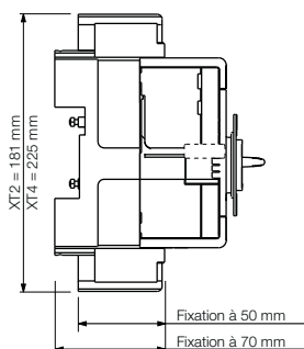
Partie fixe avec 2 adaptateurs ADP
